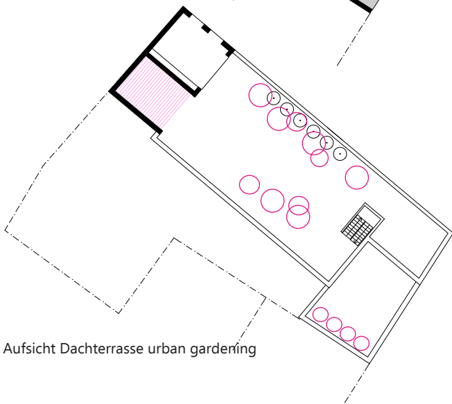
Obergeschoss Grundrissvorschlag
